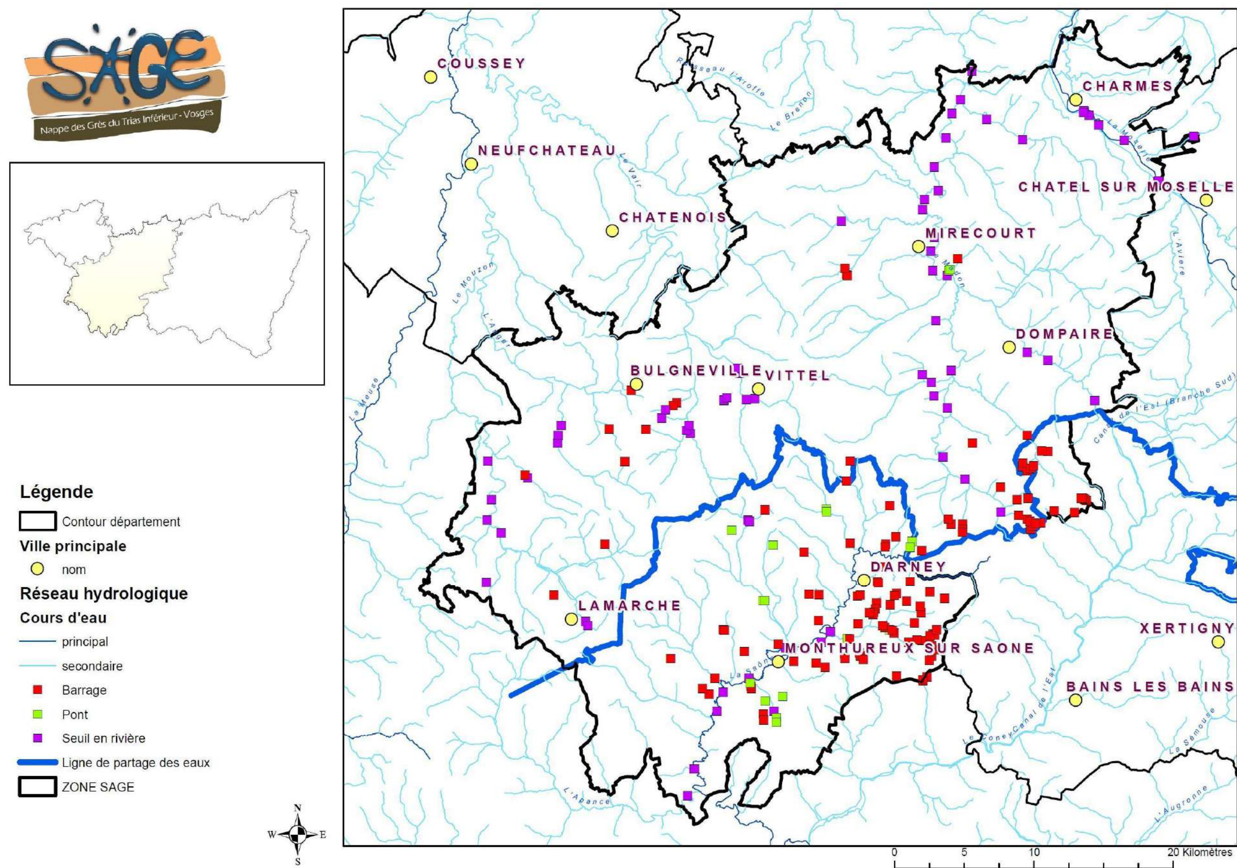
Figure 48 : Obstacles à l'écoulement recensés sur les cours d'eau du périmètre du SAGE GTI (Source : Réseau des Obstacles à l'Ecoulement - ONEMA)
